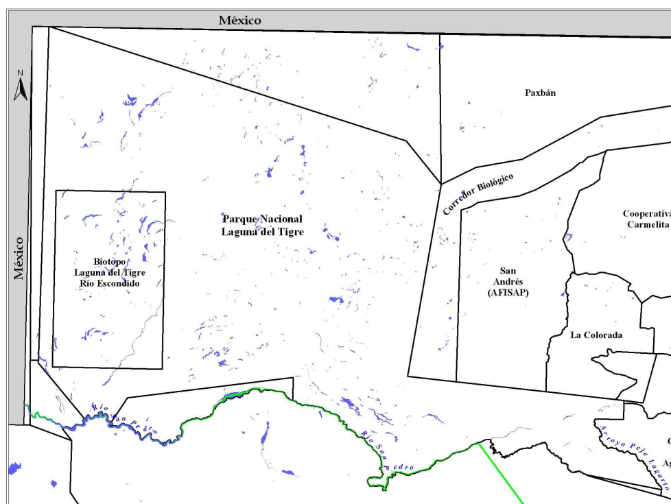
Figura No. 2: Hidrología del Parque Nacional Laguna del Tigre y Biotopo Laguna del Tigre-Río Escondido, incluyendo ríos, lagos y lagunas. (Fuente Cemec-Conap).
