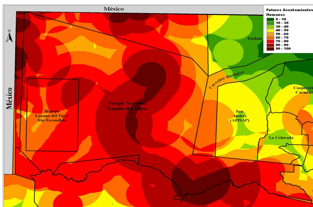
Figura No. 16: Áreas susceptibles a invasiones, futuras actividades agrícolas y ganaderas. Los colores rojos más intensos representan las áreas de mayor riesgo.
