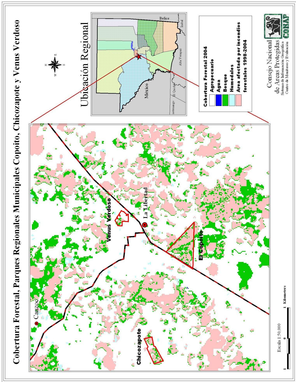
Figura 3. Cobertura forestal de los PRM de La Libertad.
